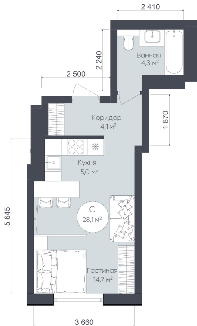
План квартиры
